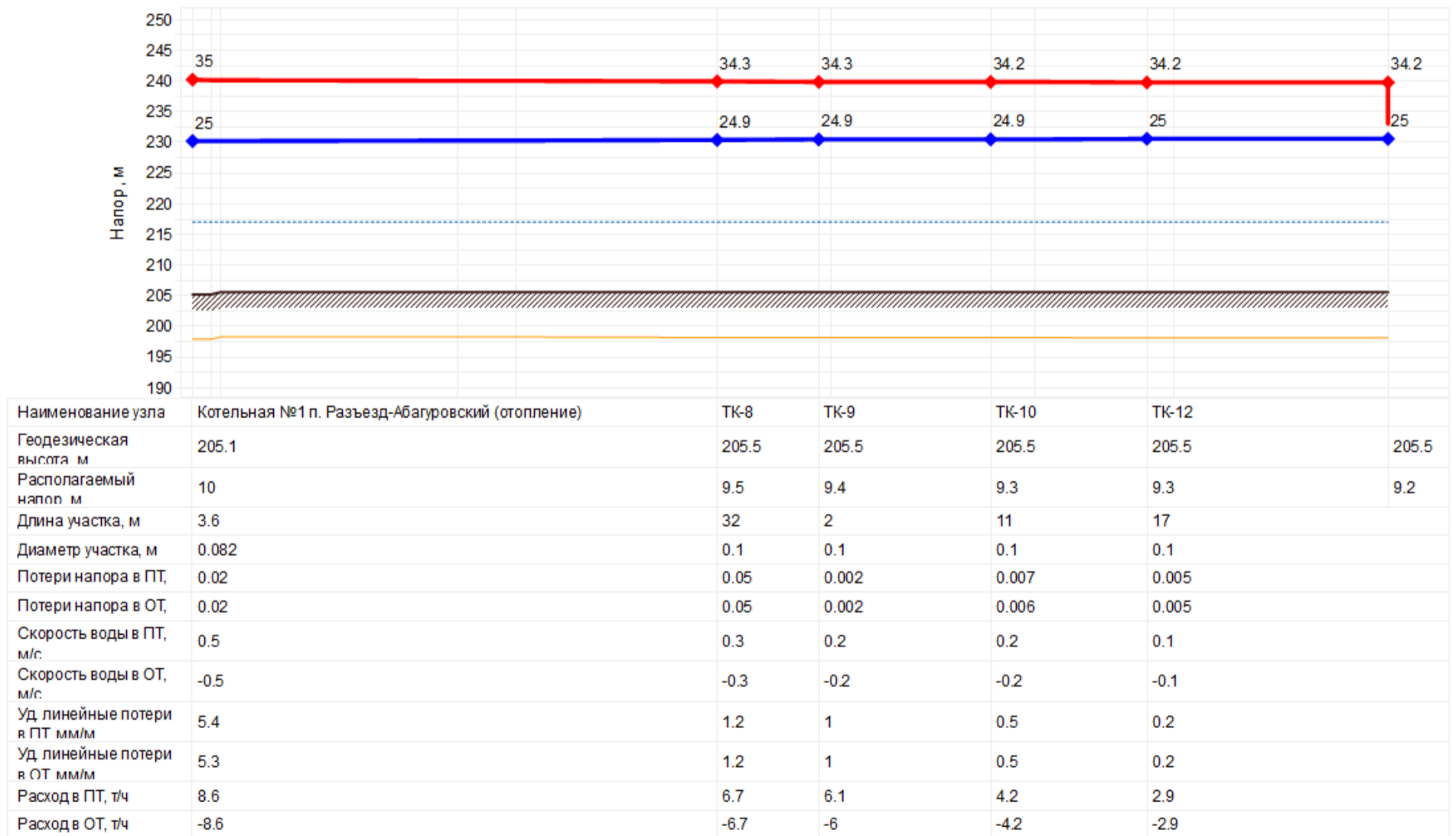
Рисунок 5.24 – Пьезометрический график магистрали Котельной №1 п. Разъезд-Абагуровский
