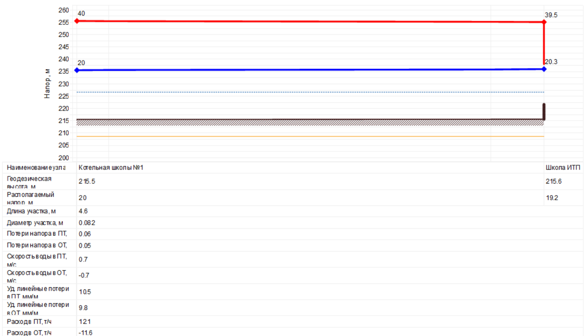
Рисунок 5.29 – Пьезометрический график магистрали Котельной школы №1
