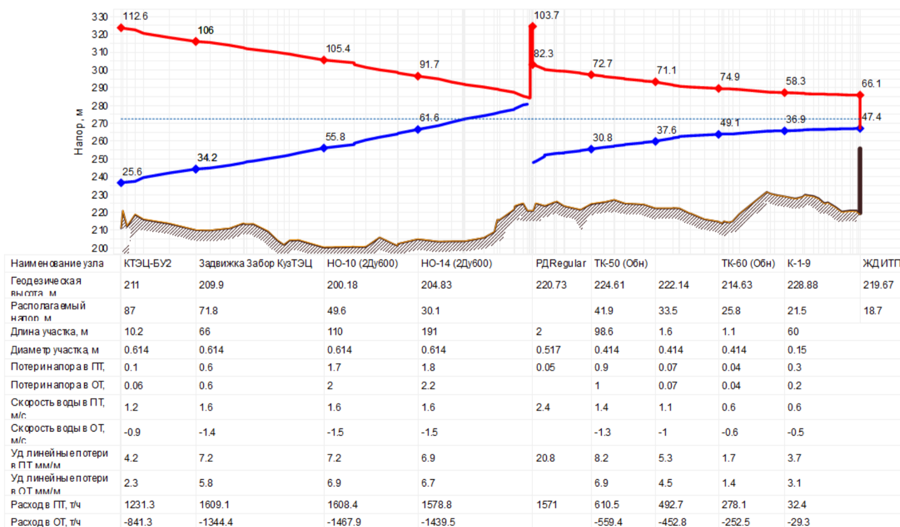
Рисунок 5.1 – Пьезометрический график магистрали КТЭЦ в Кузнецкий район
