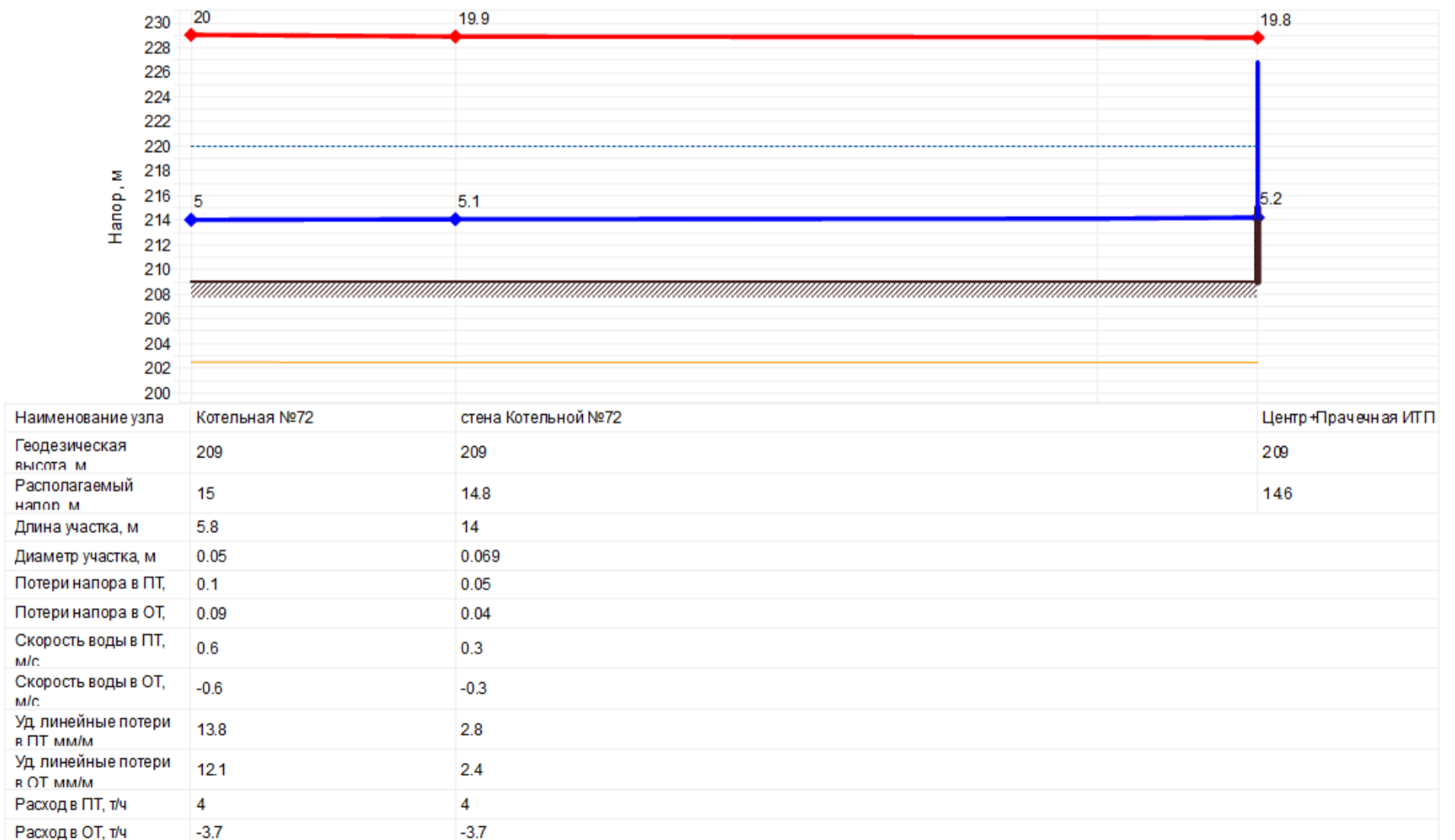
Рисунок 5.15 – Пьезометрический график магистрали Котельной №72
