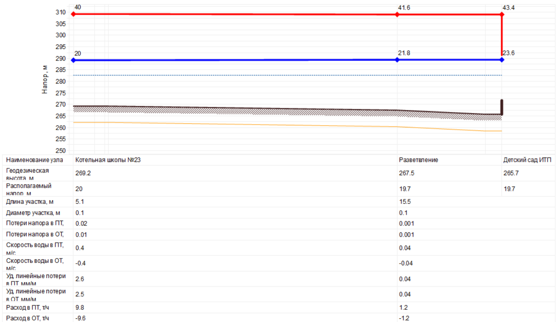
Рисунок 5.30 – Пьезометрический график магистрали Котельной школы №23
