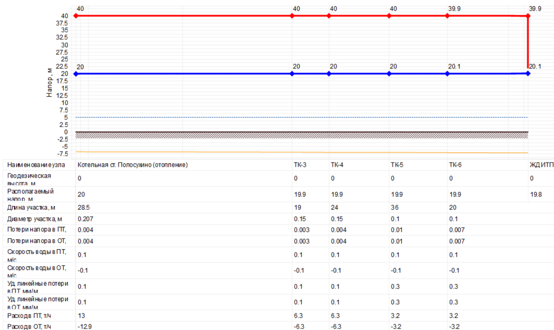
Рисунок 5.35 – Пьезометрический график магистрали Котельной ст. Полосухино
