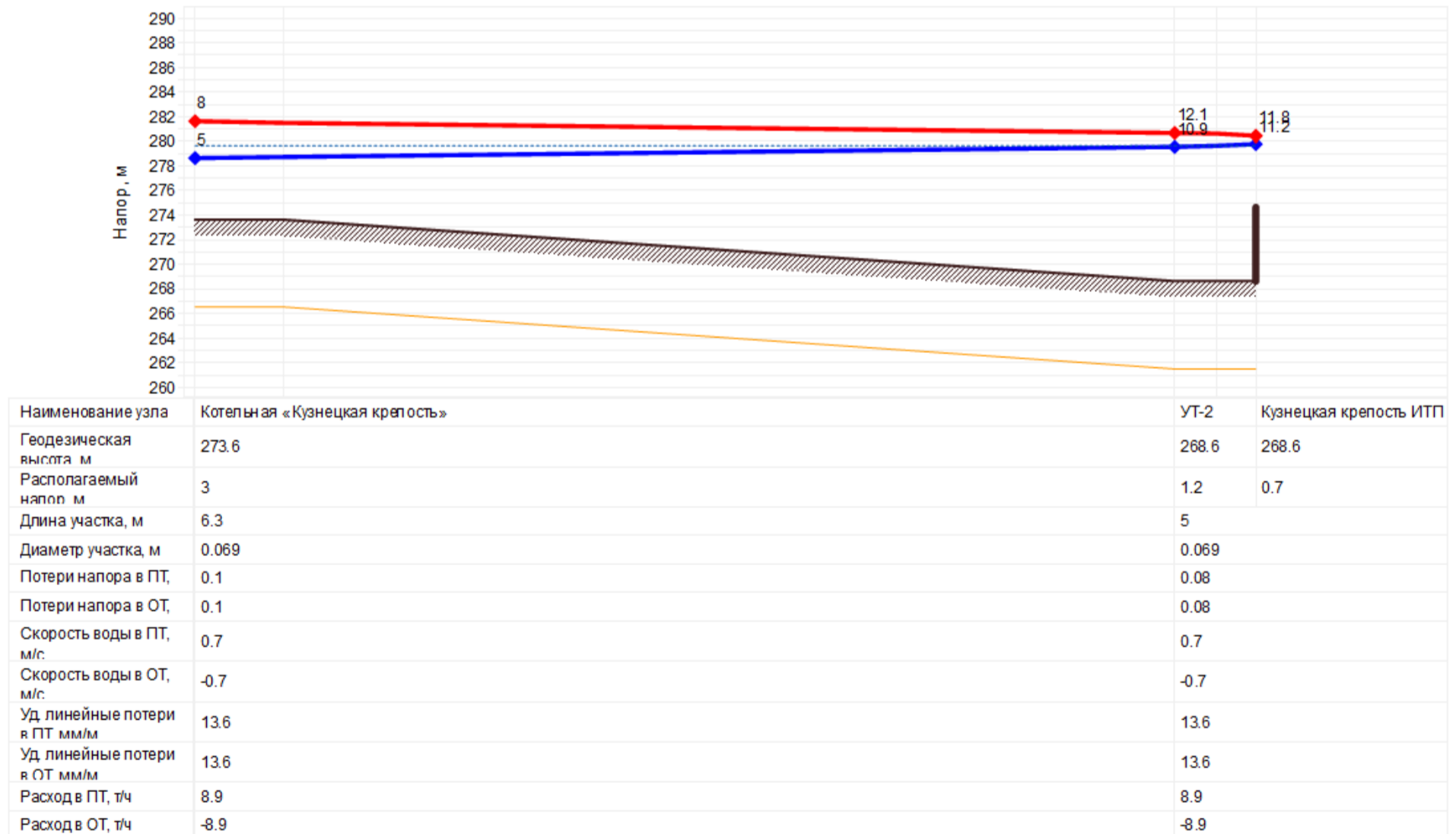
Рисунок 5.36 – Пьезометрический график магистрали Котельной «Кузнецкая крепость»
