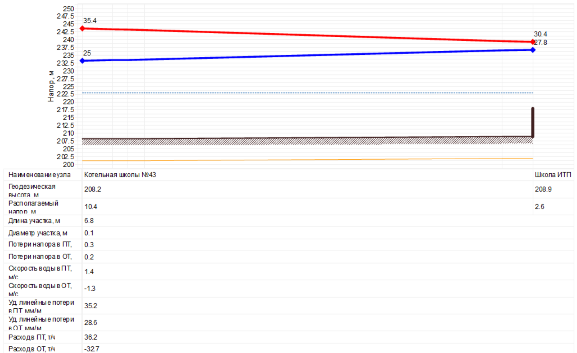
Рисунок 5.32 – Пьезометрический график магистрали Котельной школы №43
