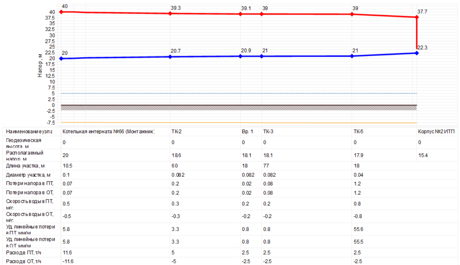
Рисунок 5.33 – Пьезометрический график магистрали Котельной интерната №66 (Монтажник)
