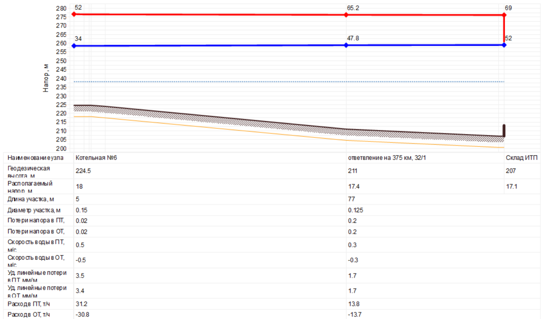
Рисунок 5.22 – Пьезометрический график магистрали Котельной №6
