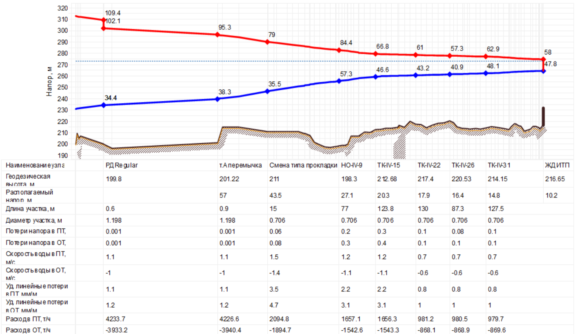
Рисунок 5.5 – Пьезометрический график Заводской магистрали ЗСТЭЦ
