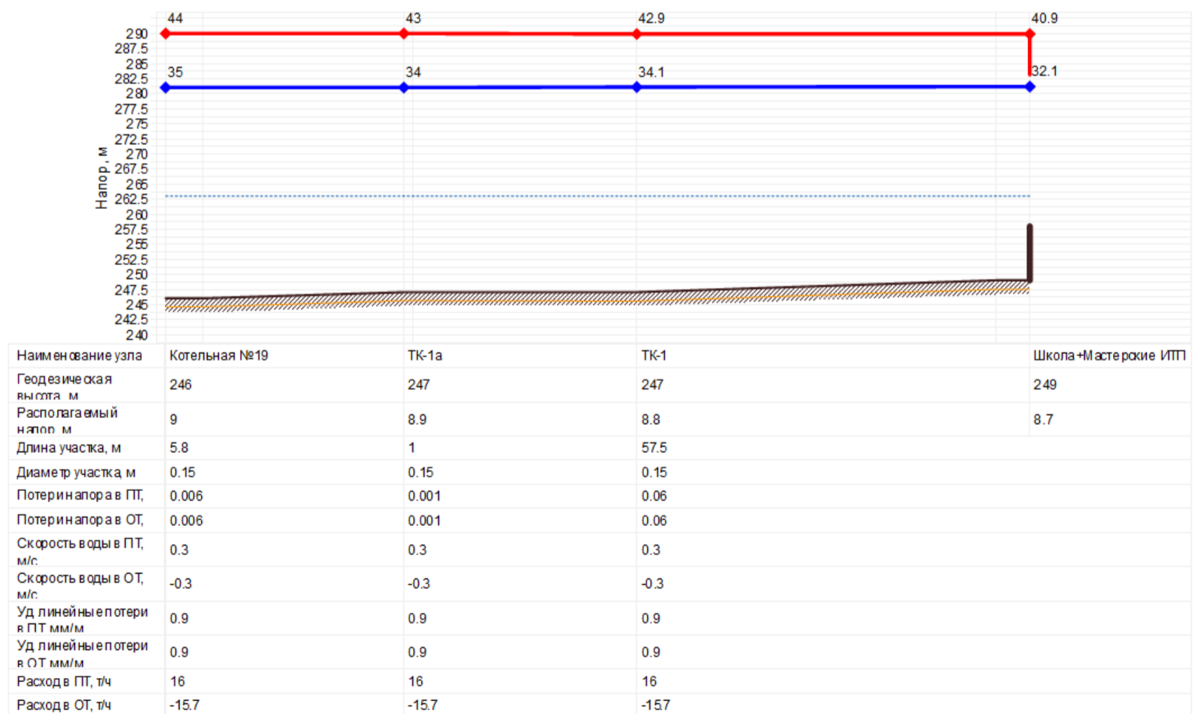
Рисунок 5.14 – Пьезометрический график магистрали Котельной №19
