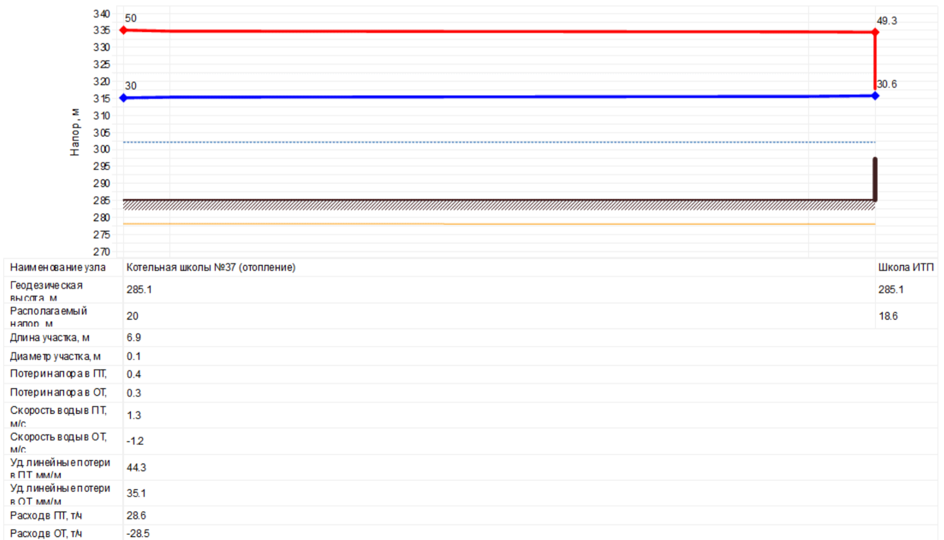
Рисунок 5.31 – Пьезометрический график магистрали Котельной школы №37
